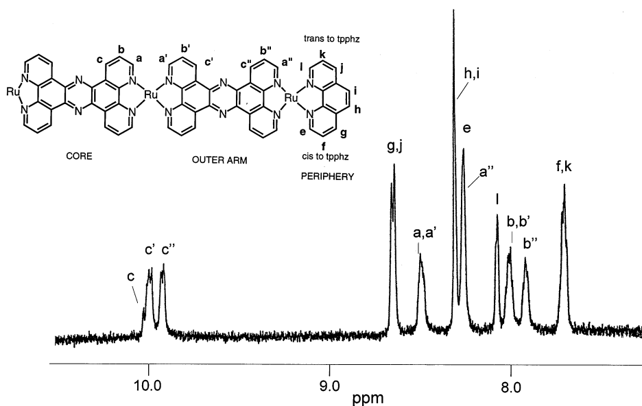
Fig. 11. ^1\text{H} -NMR Spectrum of Ru 6 [\text{PF}_6]_{12} in \text{CD}_3\text{CN} .
